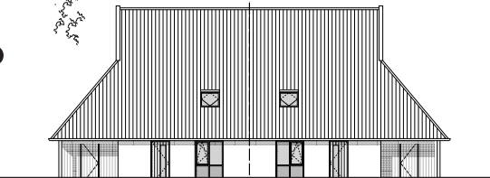
VOORGEVEL
